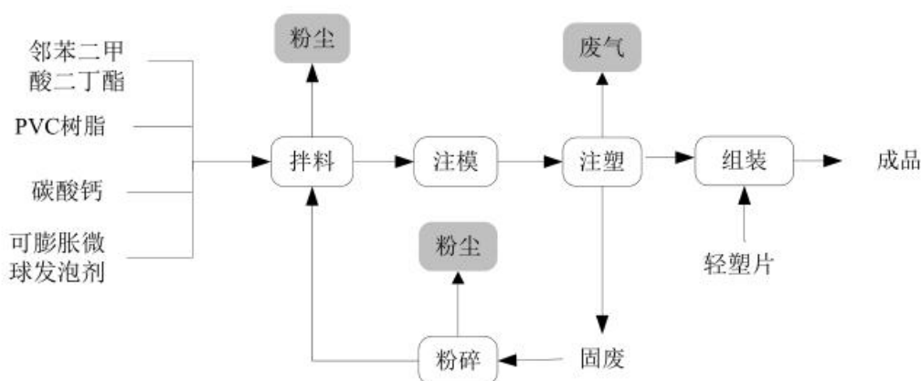
图 3-4 本项目生产工艺流程图
