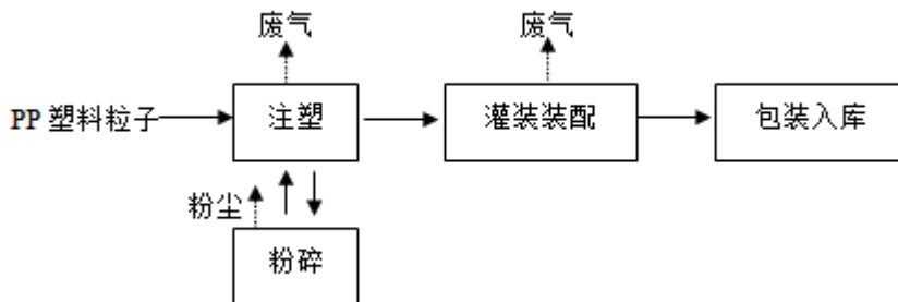
图 3-3 文具笔生产工艺及产污环节示意图
