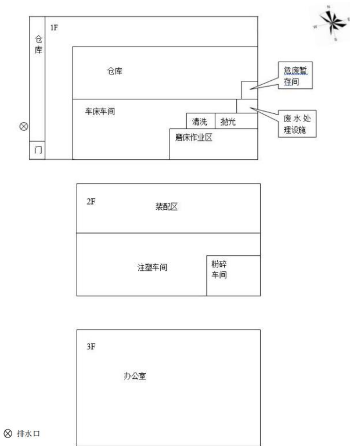
图 3-2 厂区平面布置图
