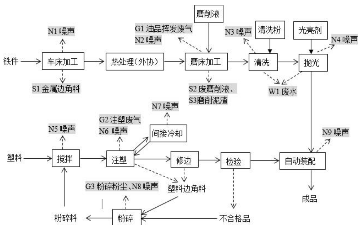
图 3-4 本项目生产工艺流程图
