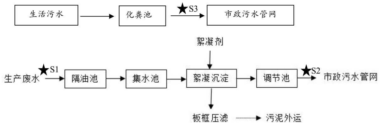
图 4-1 废水处理工艺流程图
