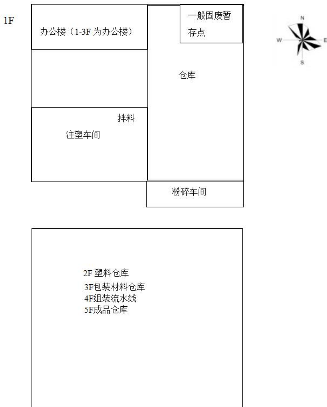
图 3-2 厂区平面布置图 (1 厂区)
