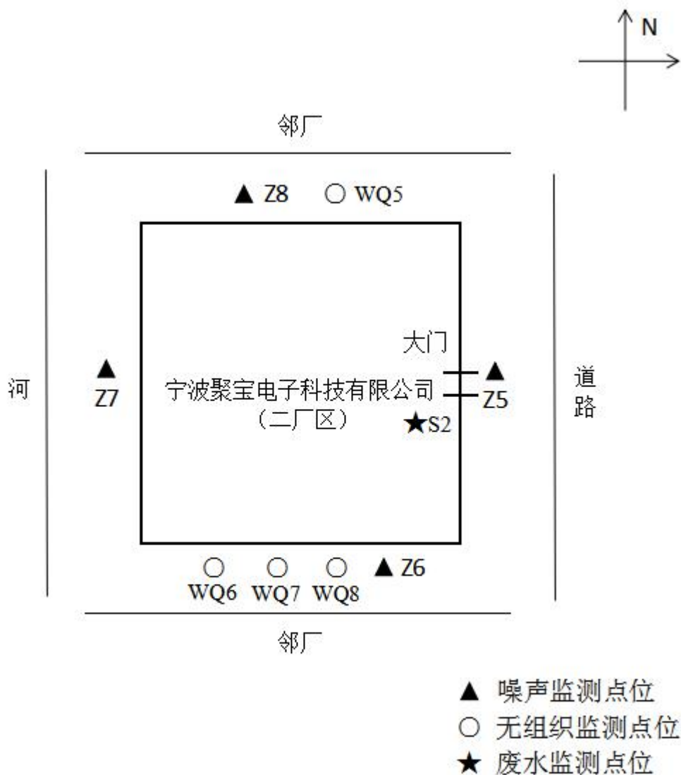
图 7-1 监测点位图 (2 厂区)
