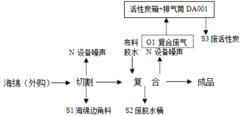
图 3-3 本项目生产工艺流程图
