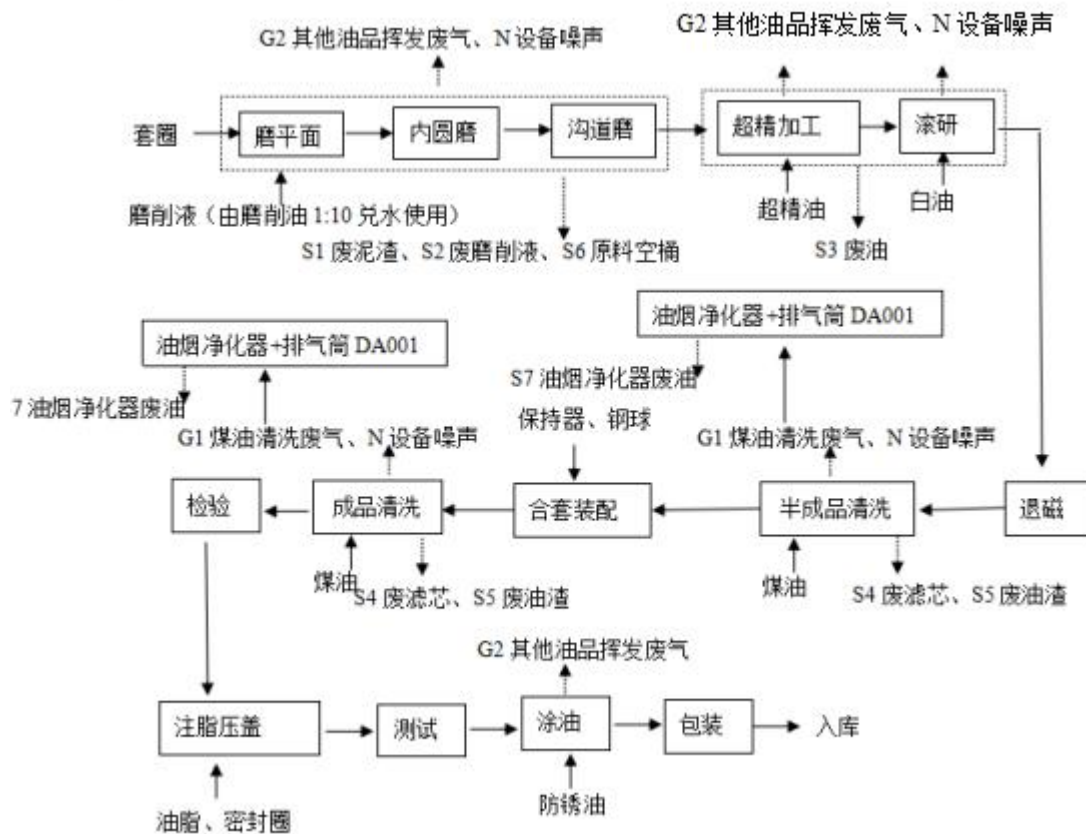
图 3-3 本项目轴承生产工艺流程图
