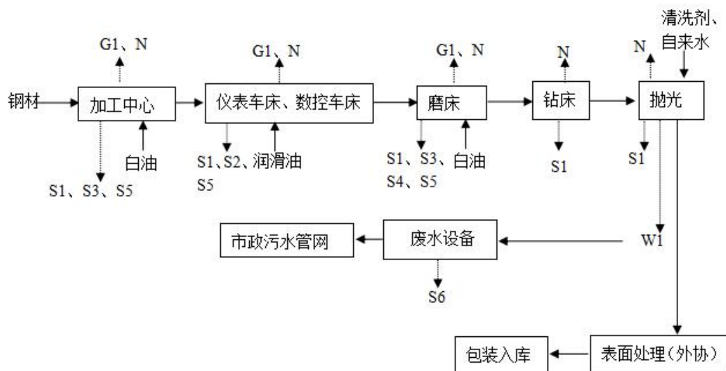
图 3-3 本项目生产工艺流程图
