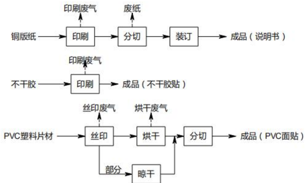
图 3-3 生产工艺及产污节点图
