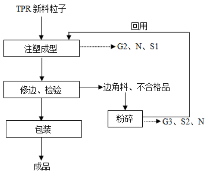
图 3-3 TPR 鞋底生产工艺流程图
