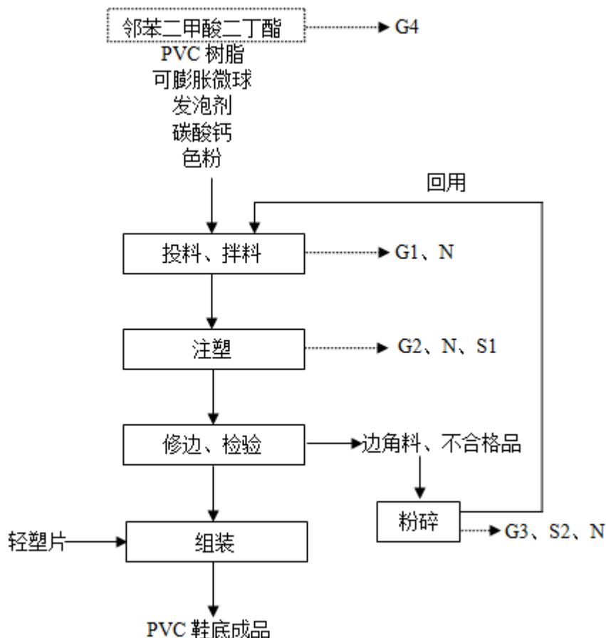
图 3-2 PVC 鞋底生产工艺流程图
