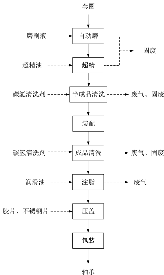
图 2-1 本项目生产工艺流程图
