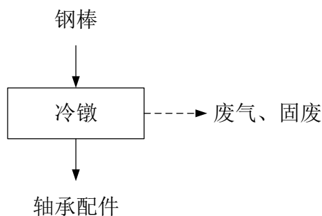
图 2-1 本项目生产工艺流程图
