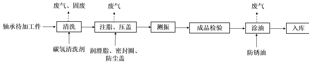
图 2-2 本项目生产工艺流程图
