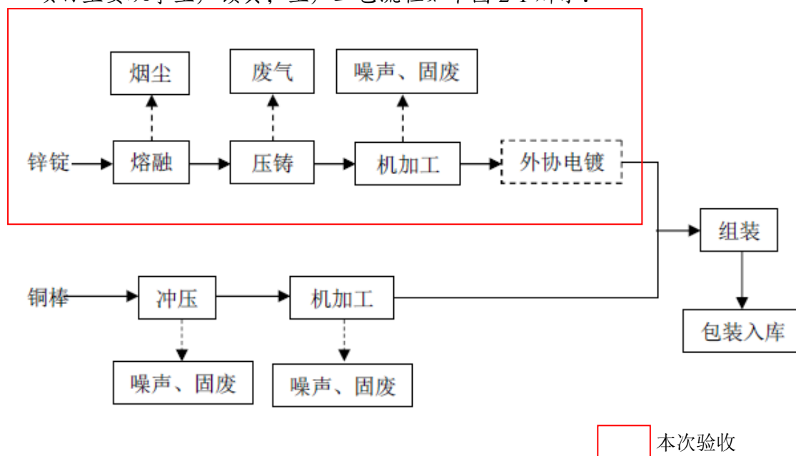
图 2-1 本项目生产工艺流程图
