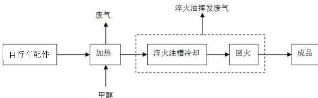
图 2-1 本项目生产工艺流程图
