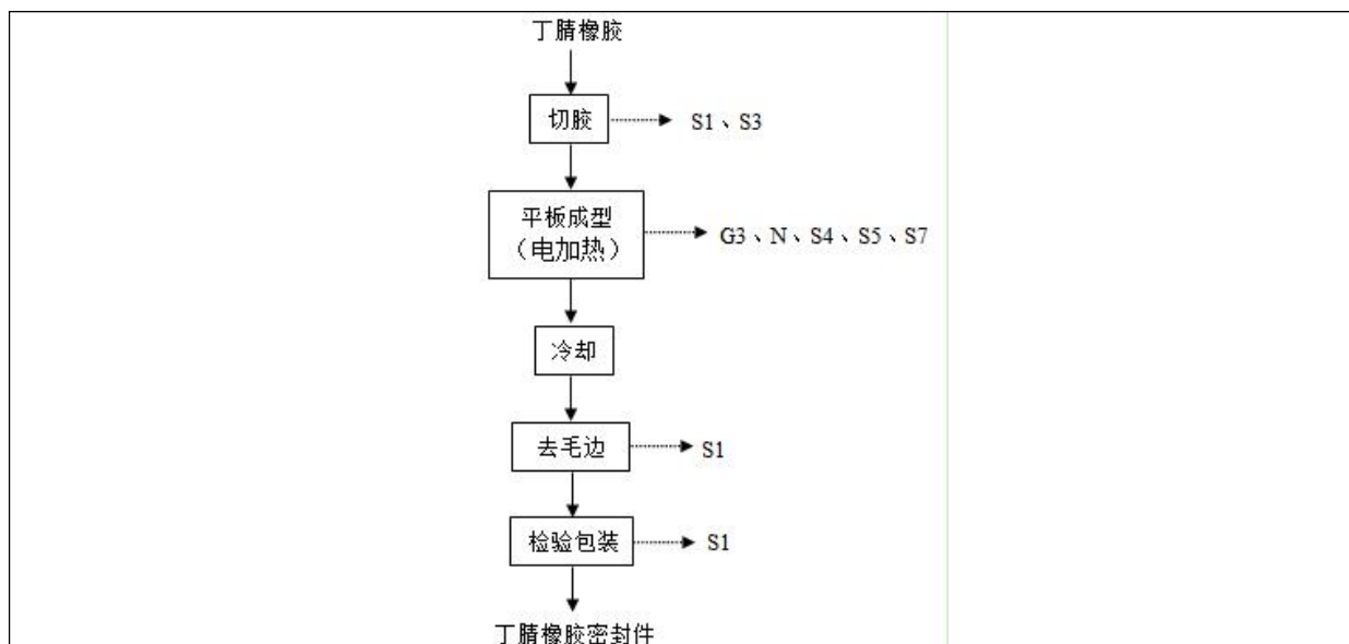
图 2-2 本项目丁腈橡胶密封件工艺流程图
