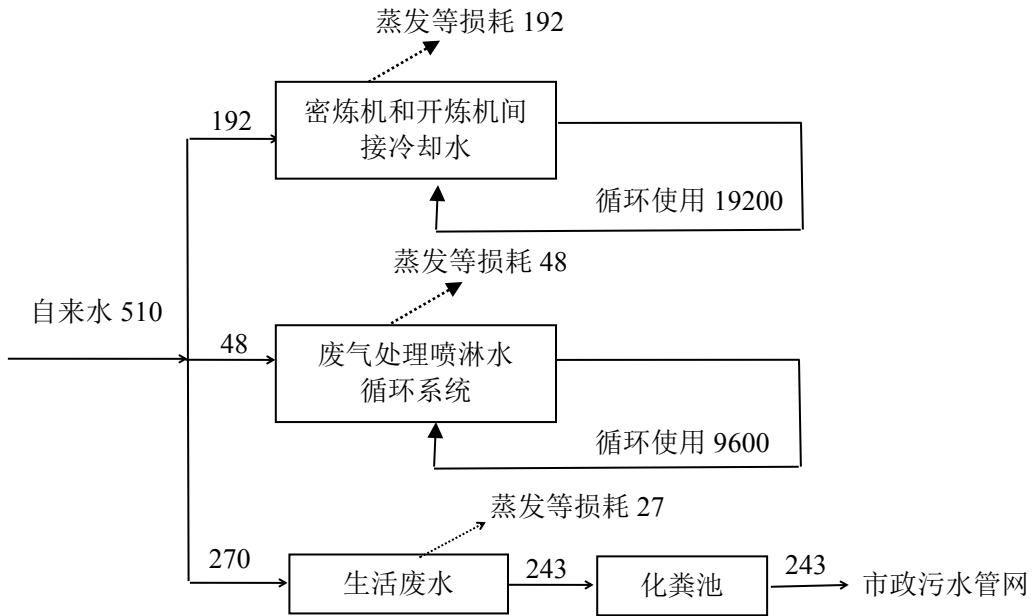
图 2-1 项目第一阶段水平衡图 (单位: t/a)
