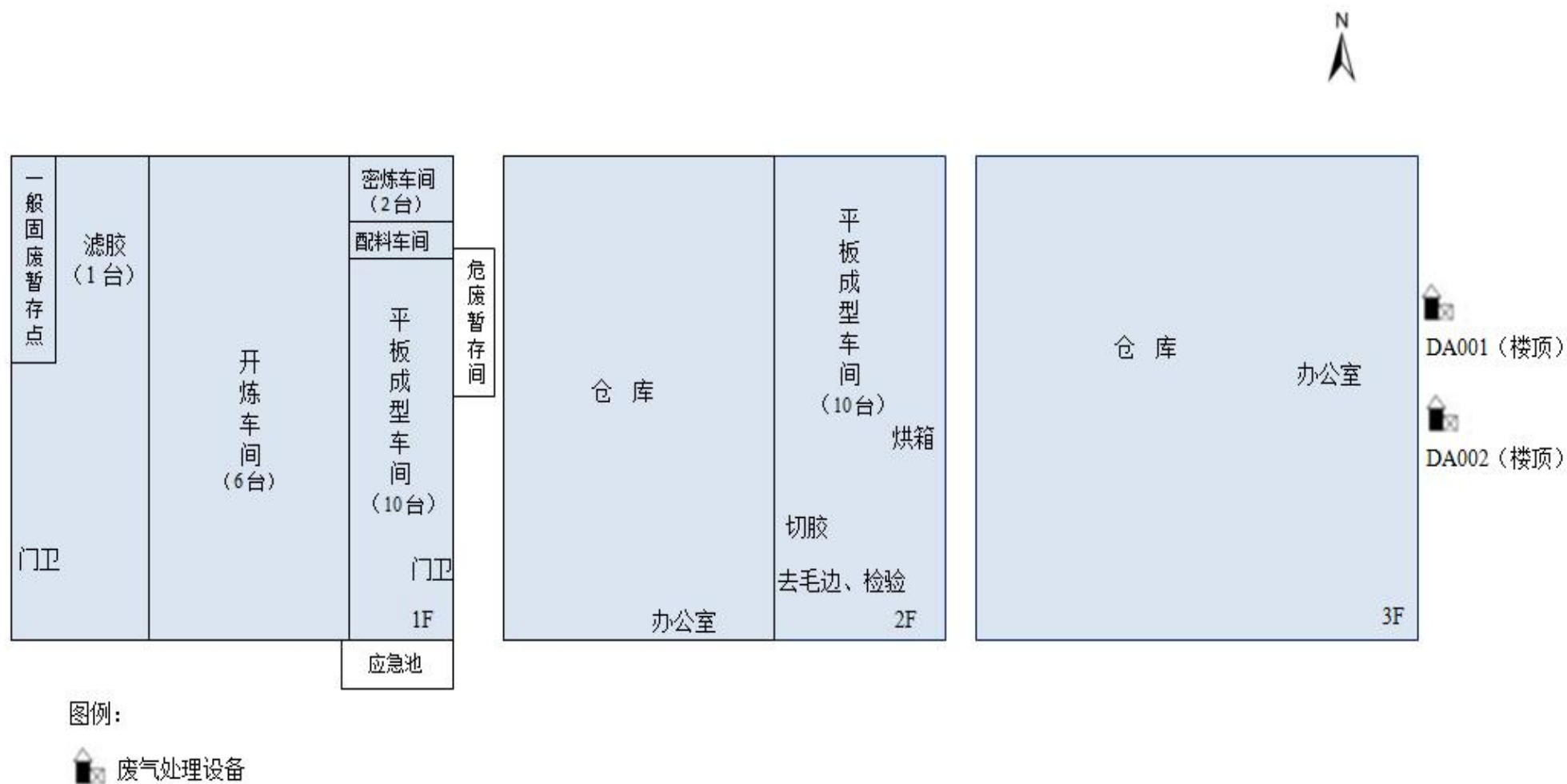
附件3 厂区平面布置图
